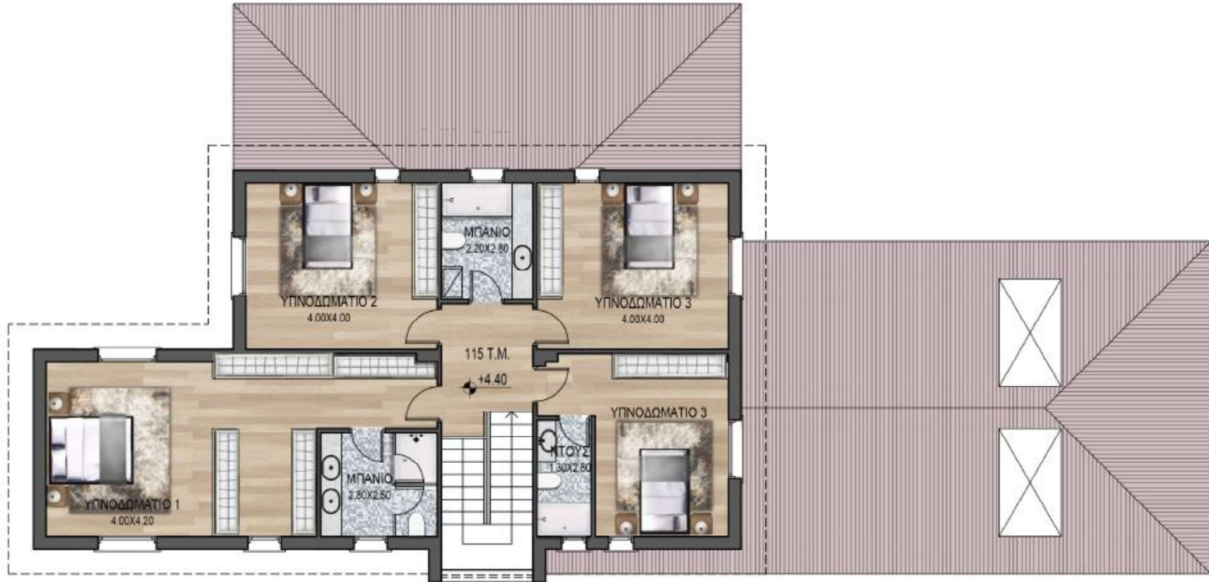
ΚΑΤΩΨΗ ΟΡΟΦΟΥ
