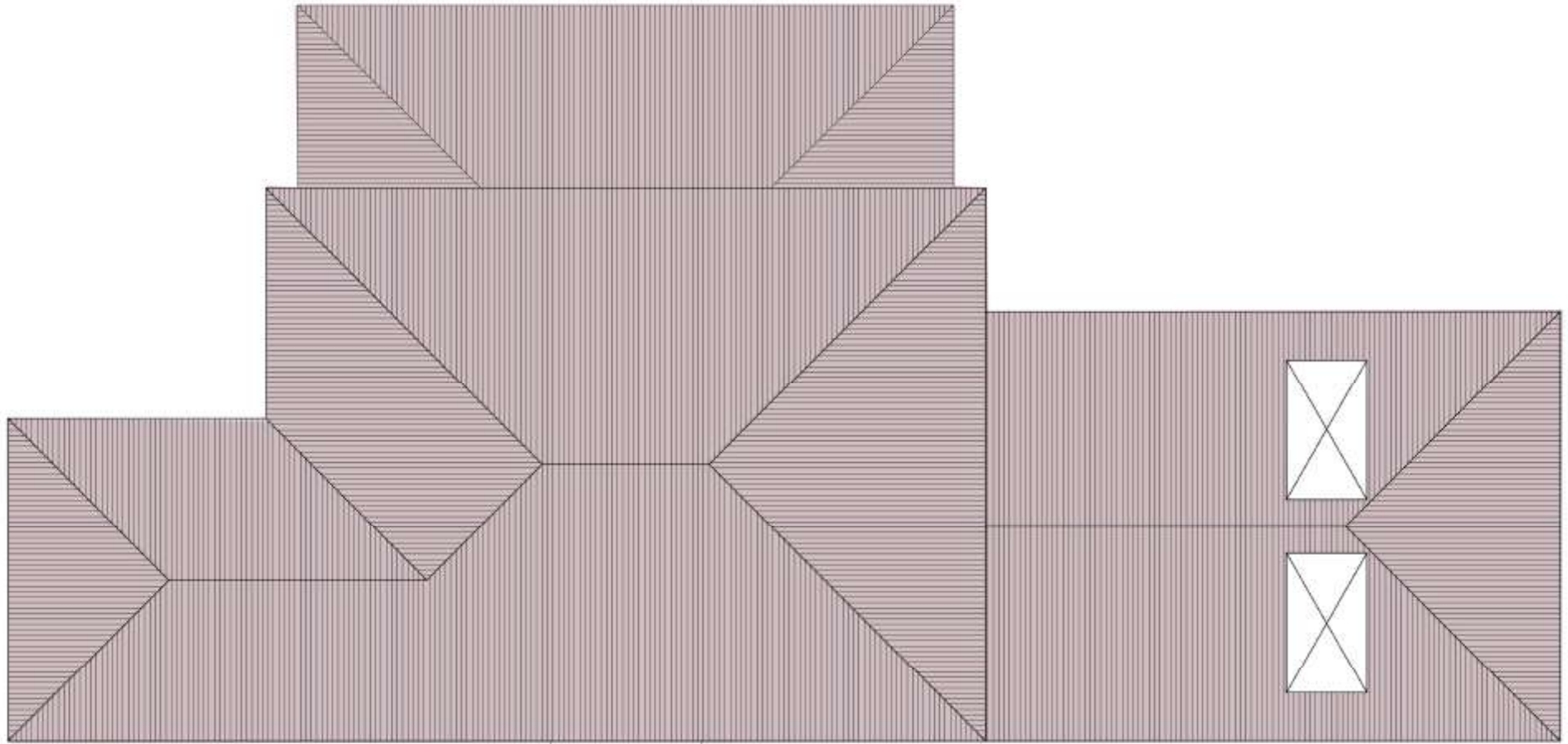
ΚΑΤΟΨΗ ΟΡΟΦΗΣ
